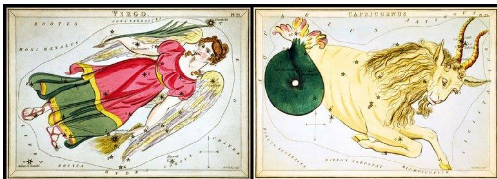
Figur 1. Stjärnbilderna Jungfrun och Stenbocken.
