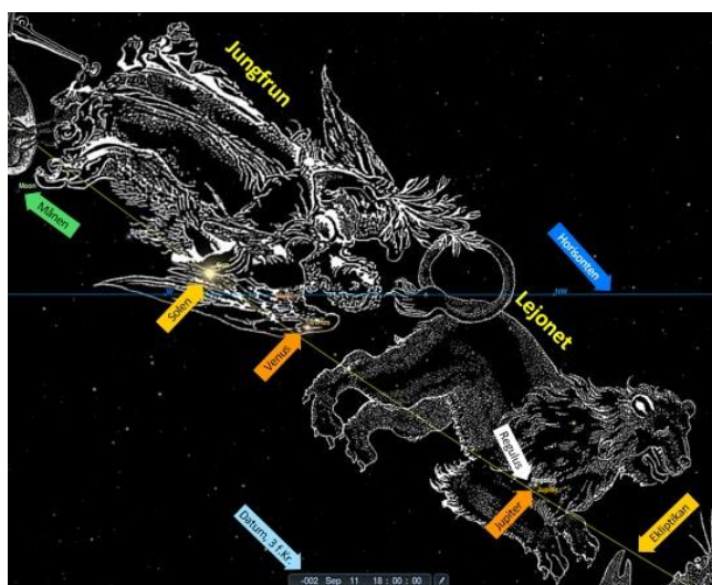
Figur 2. Stjärnhimlen sedd västerut från Jerusalem vid Jesu födelse. Blå linje är horisonten (marken är borttagen för tydlighet). Gul linje är ekliptikan utmed vilken sol, måne och planeter rör sig. (År "-2" innebär år "3 f.Kr." eftersom år 0 inte finns i vår gregorianska tideräkning men däremot i planetarierna.)
