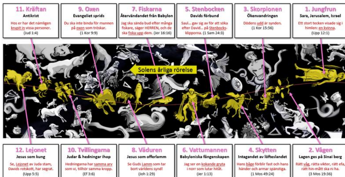
Figur 3. Sammanfattning av frälsningshistorien på himlen. De gula stjärnbilderna utmed ekliptikan (vågad linje) är dem i Mazzaroten.
